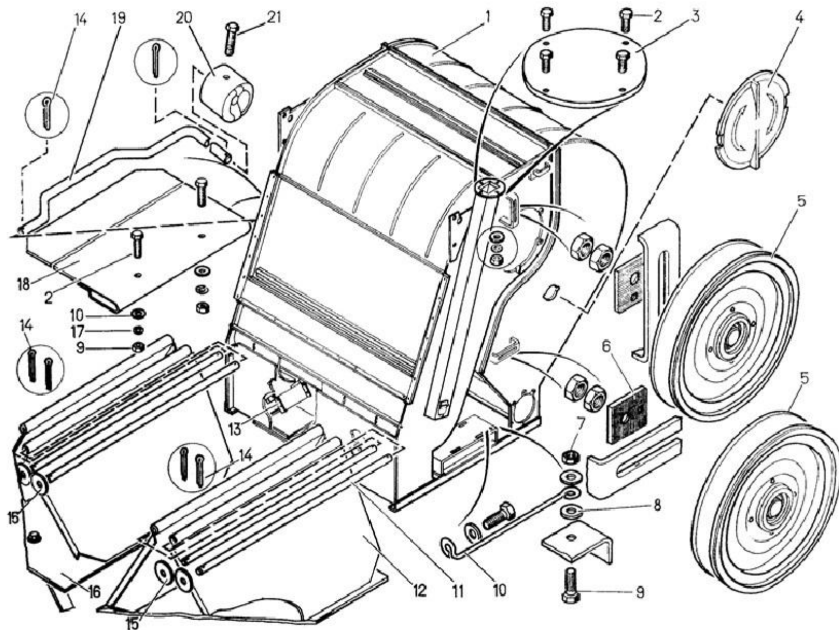
МПО 50.04.000. Воздушная часть
